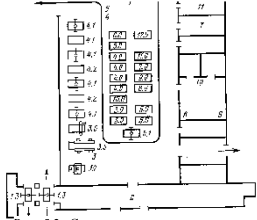
Рис. 5.2. Схема расположения постов и участков типовой СТОА. I - производственная зона; II - административная зона.
