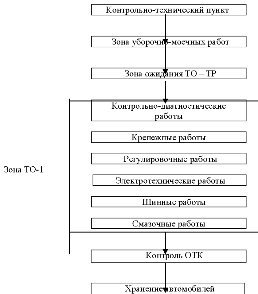
Рис.5.1.Схема технологического процесса ТО-1 автомобилей
