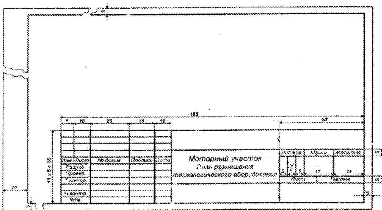
Основная надпись по ГОСТ 2.104-68 (угловой штамп), который проставляется в правом нижнем углу формата А1 графической части проекта.
