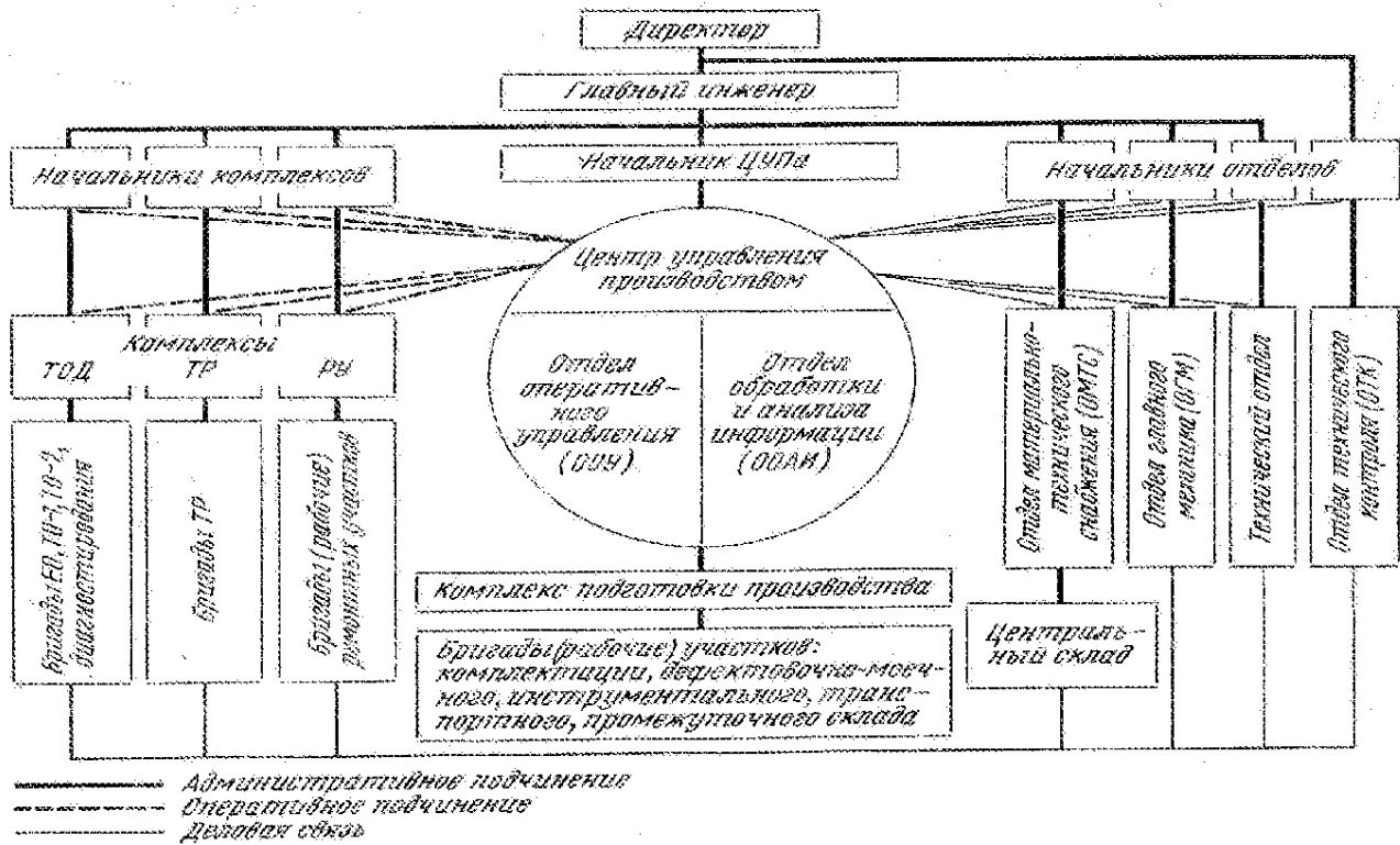
Рис.4.1. Структура централизованного управления технической службой АТП
