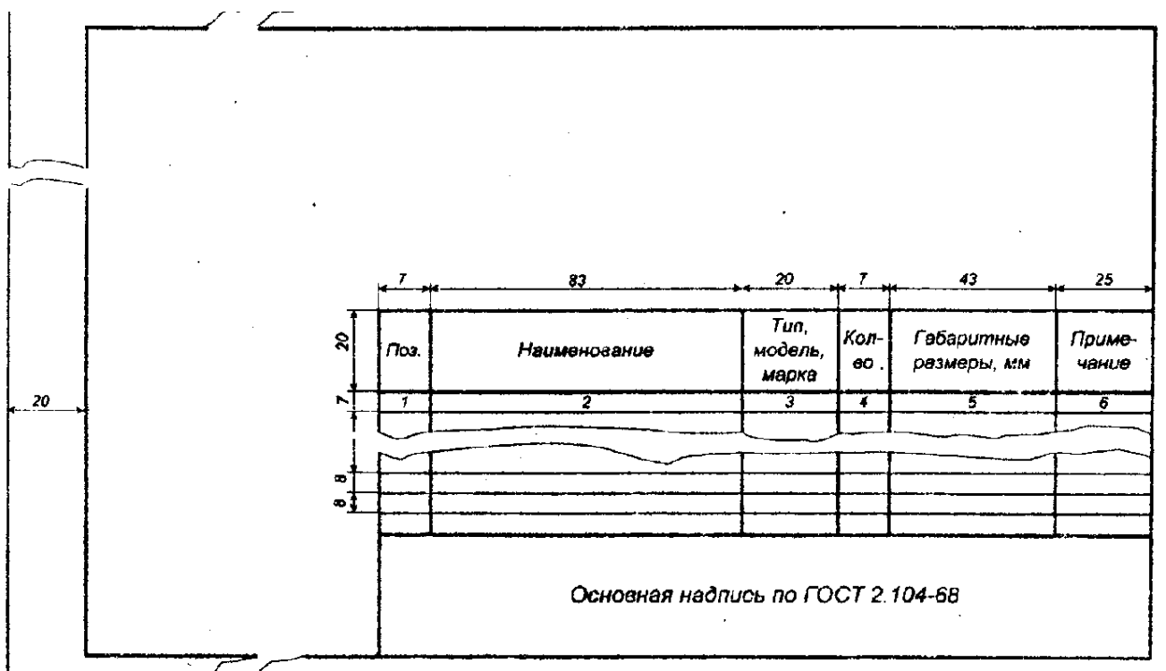
Спецификация технологического оборудования и организационной оснастки. Выполняется над основной надписью (угловым штампом) на листе формата А1
