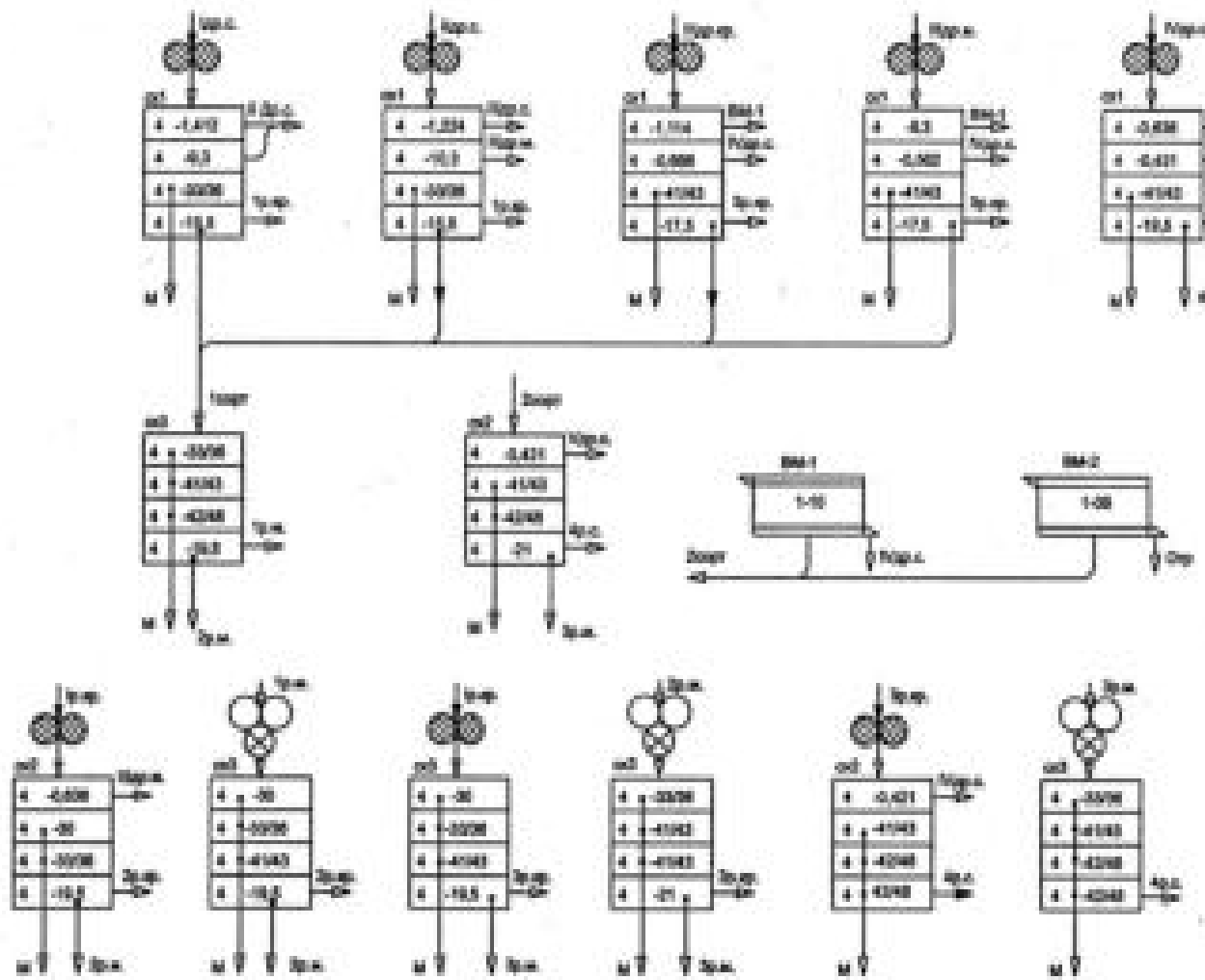
Примерная технологическая схема 63 % помола ржи в сеяную муку
