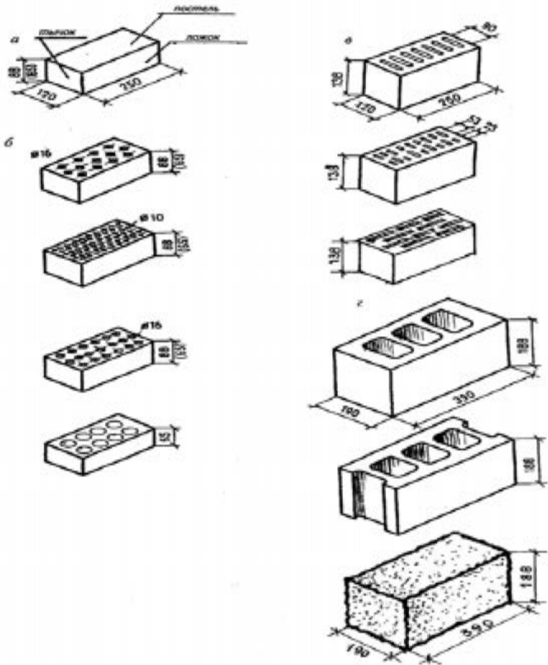
Рис. 12. Стеновые изделия из искусственных каменных материалов: а – полнотелые керамические и силикатные кирпичи; б – тоже, эффективные многодырчатые и облицовочные в) – керамические блоки с щелевыми пустотами; г – бетонные стеновые блоки – пустотные из керамзитобетона и сплошные из ячеистых бетонов.
