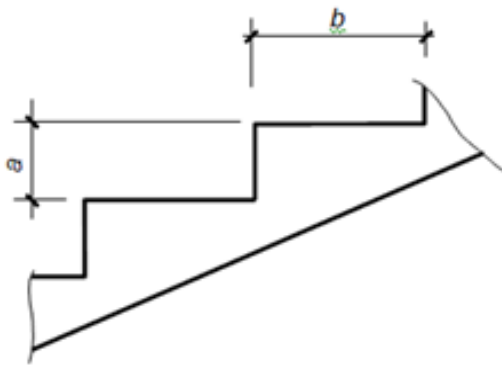
Рис. 4. Элементы лестничного марша: а - подступенок, в - проступь.
