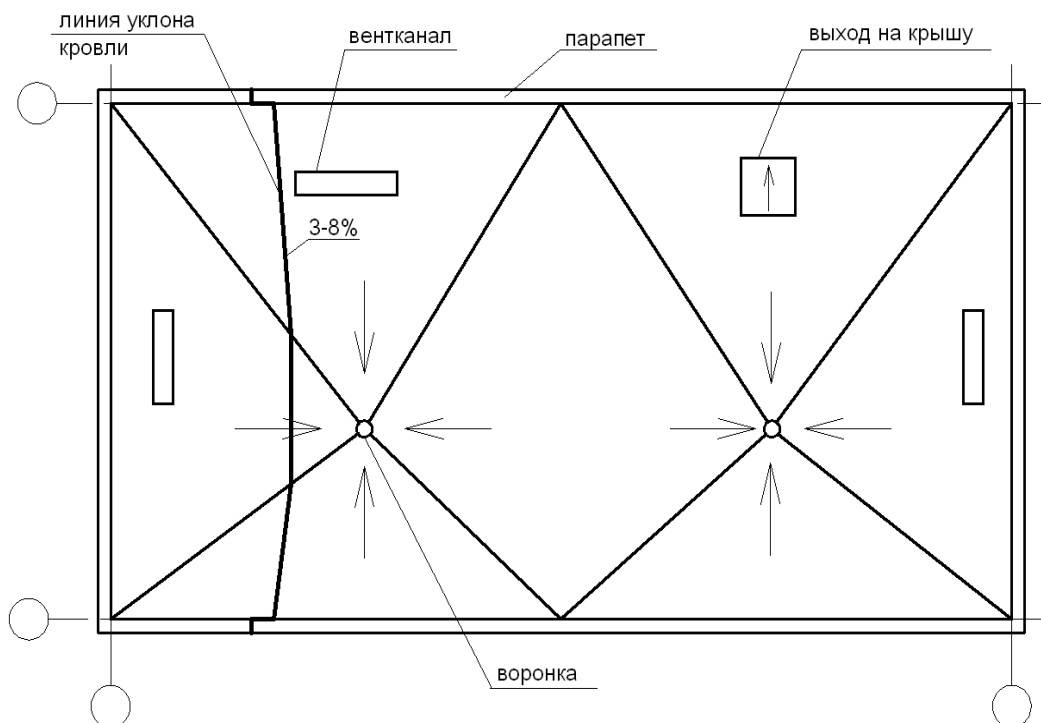
Рис. 16. Пример изображения плана плоской крыши малоэтажного жилого здания
