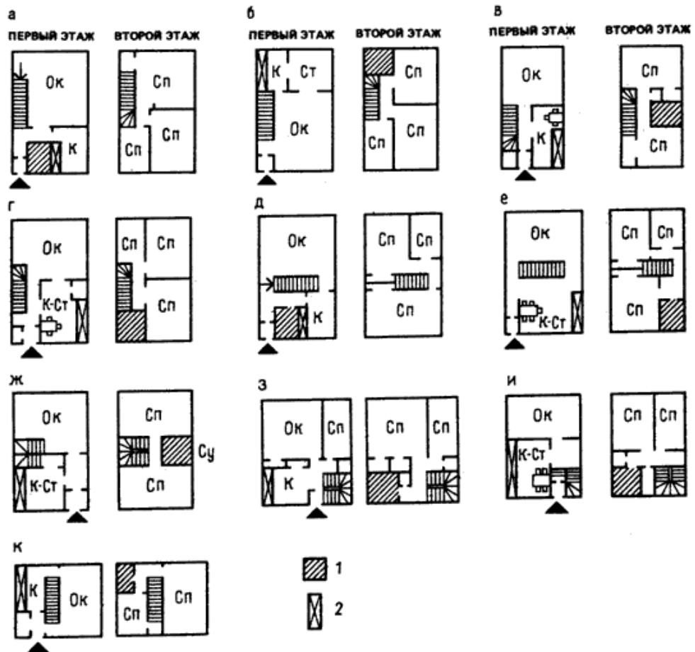
Рис. 7. Планировочные решения двухуровневых квартир при различных вариантах размещения внутриквартирной лестницы. Условные обозначения: 1 – санузел; 2 – кухонное оборудование; Ок – общая комната; Сп – спальня; К – кухня; К-Ст – кухня-столовая.
