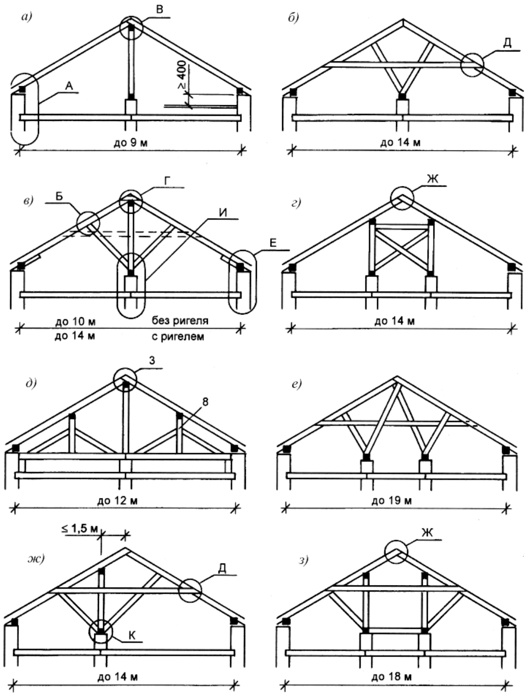
Рис. 17. Стропильные конструкции двухскатных крыш.
