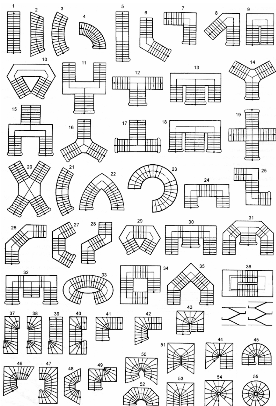
Рис. 6. Варианты лестниц по форме маршей и площадок, по количеству маршей, по форме ступеней:
