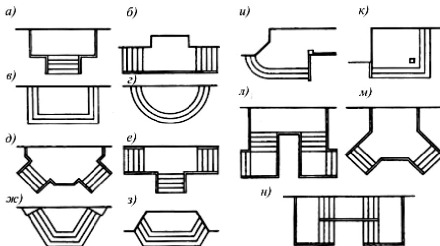
Рис. 8. Варианты планировочных решений наружных, входных площадок со ступенями.
