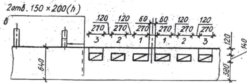
Рис. 20. Примеры изображения вентиляционных каналов на плане
