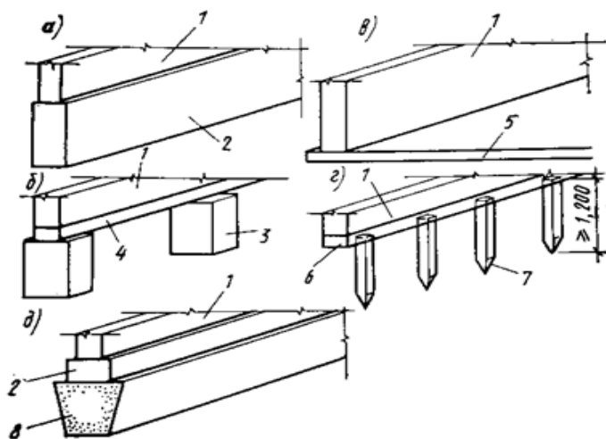
Рис.13. Конструктивные схемы фундаментов малоэтажных жилых зданий: а - ленточный фундамент; в - столбчатый; в - плитный; г - фундамент на коротких сваях; д - ленточный фундамент на песчаной подушке; 1 – стена; 2 – лента фундамента; 3 столб; 4 – фундаментная балка; 5 – монолитная железобетонная плита; 6 - ростверк; 7 – свая; 8 – песчаная подушка.
