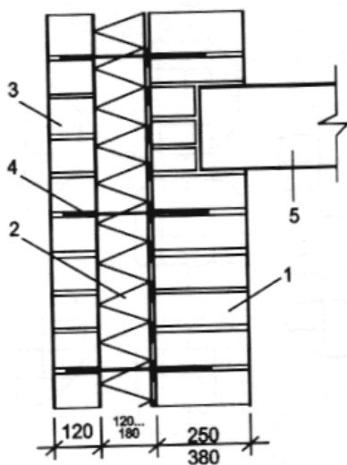
Рис. 10. Стена с облицовочным самонесущим слоем из кирпича: 1– несущий слой кладки; 2– плитный утеплитель; 3– облицовочный слой кладки; 4– гибкая связь; 5 – плита перекрытия.
