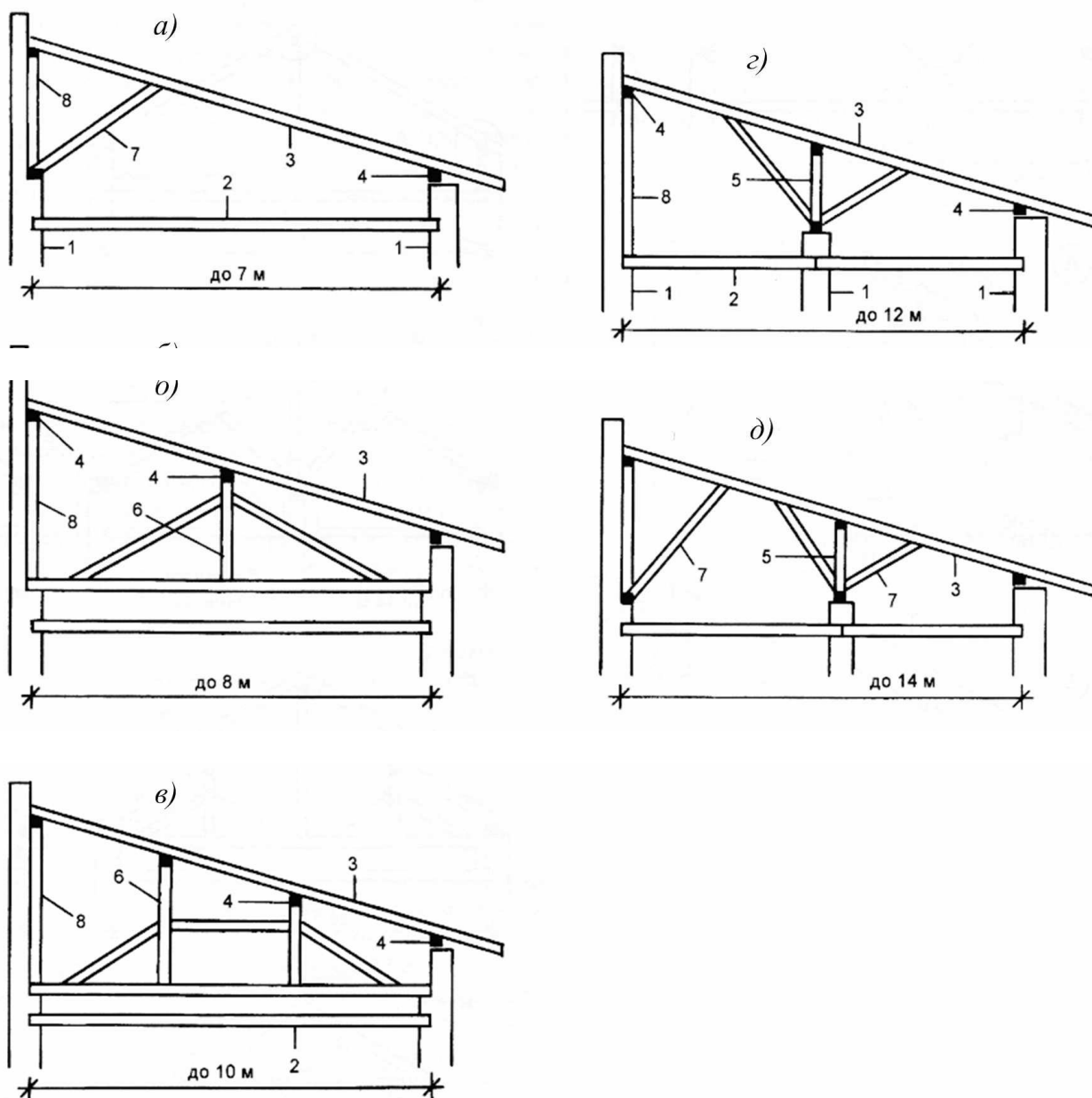
Рис. 20. Стропильные конструкции односкатных крыш: 1 – стена; 2 – перекрытие; 3 – стропило; 4 – подстропильный брус; 5 – стойка; 6 – стойка шпренгеля; 7 – подкос; 8 – пристенная стойка
