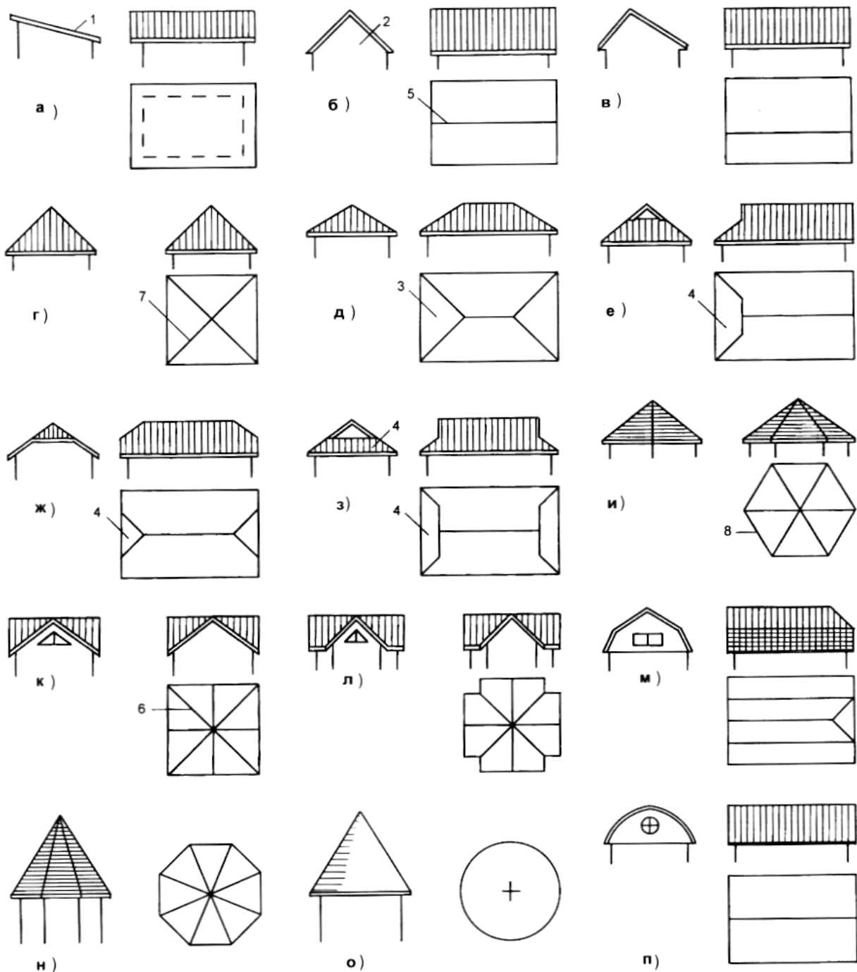
Рис.14. Основные формы и элементы скатных крыш:
