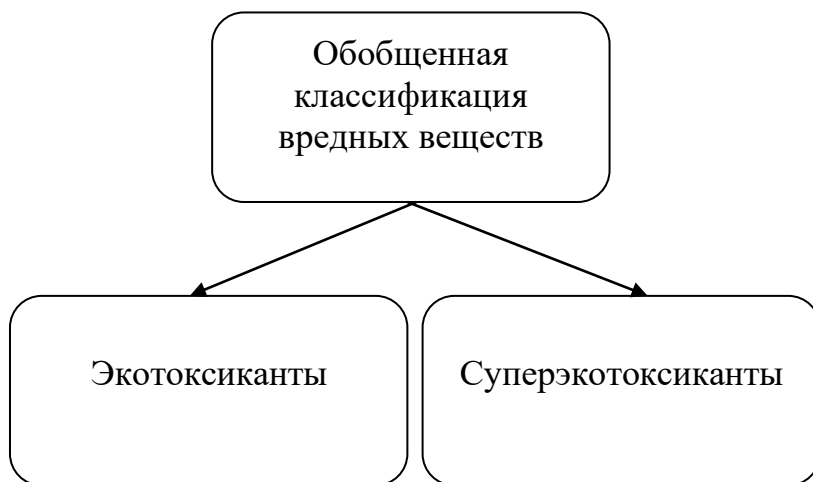
Рис. 2. Экотоксиканты и суперэкотоксиканты
