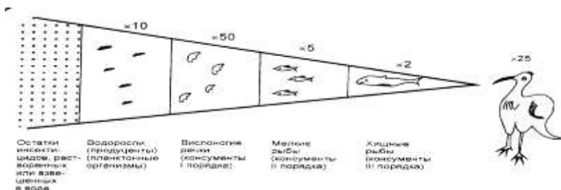
Рис. 8. Биоаккумуляция инсектицида ДДТ в водных объектах
